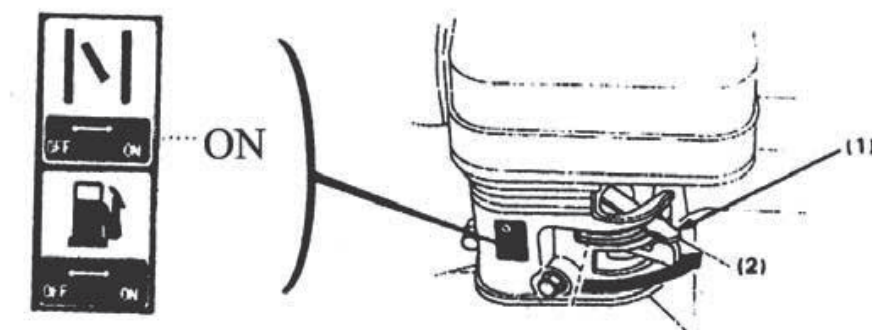
(1) dźwignia ssania (2) "ON"
