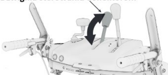
Dźwignia sterowania deflektorem
